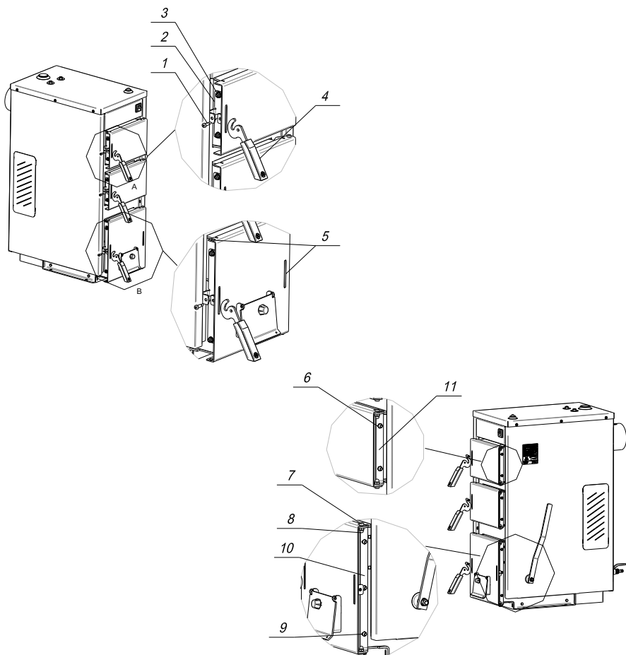
Rysunek 6. Zmiana kierunku otwierania drzwiczek
