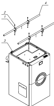
Rys. 2. Schemat ideowy przenoszenia kotła
