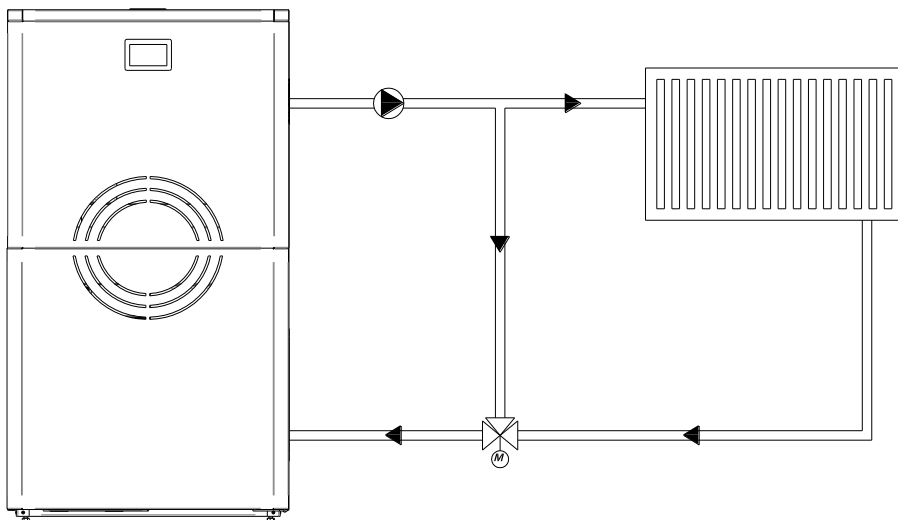
Rys. 4a. Schemat montażu zaworu trójdrożnego w celu ochrony temperatury powrotu
