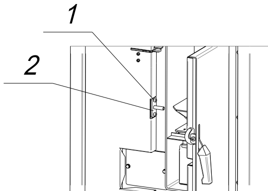
Rys. 10. Schemat regulacji zaczepek drzwiczek kotła
