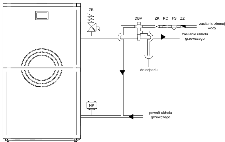
Rys. 4e. Przykładowy schemat zabezpieczenia instalacji ogrzewania wodnego, wg normy PN-EN 12828
